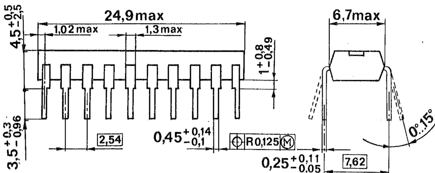
Bild 7 (DIP-18, Keramik)
