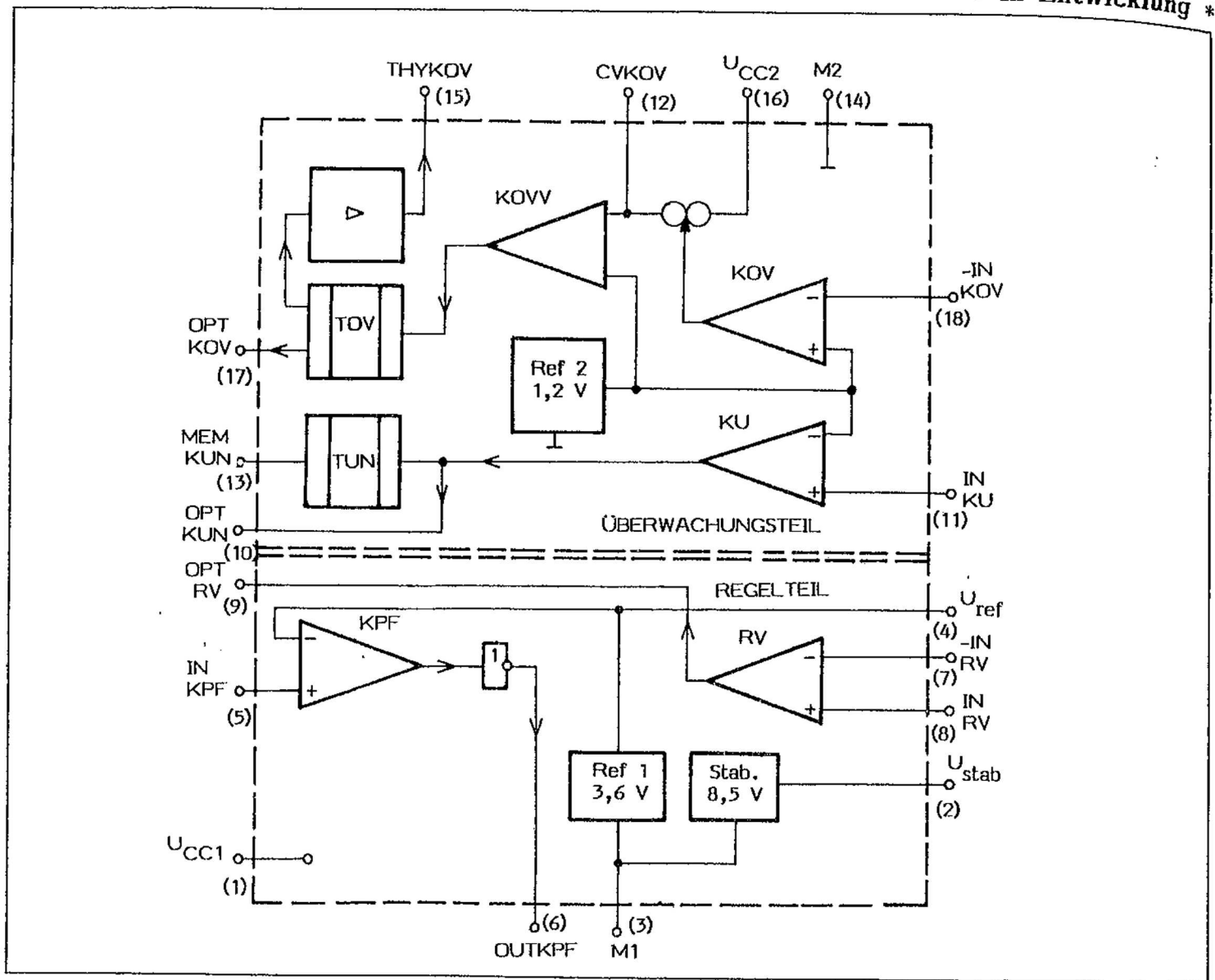
Übersichtsschaltplan
